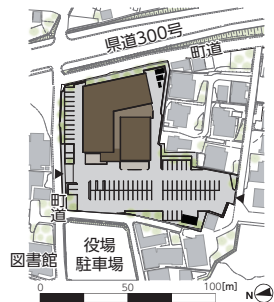
配置図
